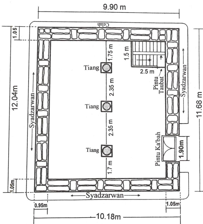
Gambar pondasi Ka'bah, pintu Taubat, serta tiang-tiang di dalam Ka'bah
